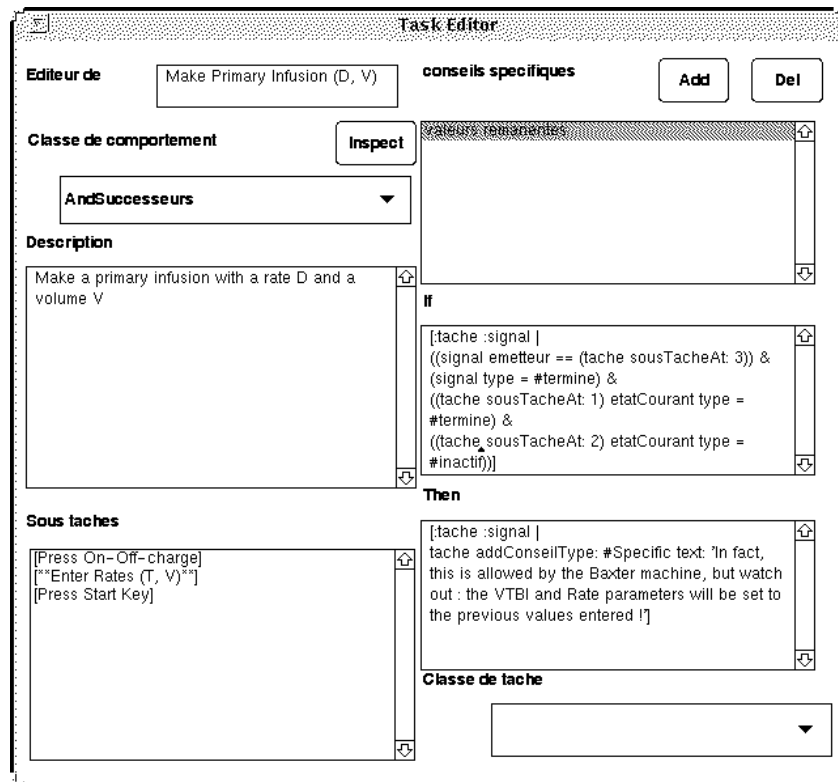
Figure 5: Éditeur de tâche pour l'exemple de l'infusion primaire, avec conseil spécifique.
