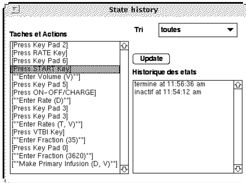
Figure 8. Historique des états.
