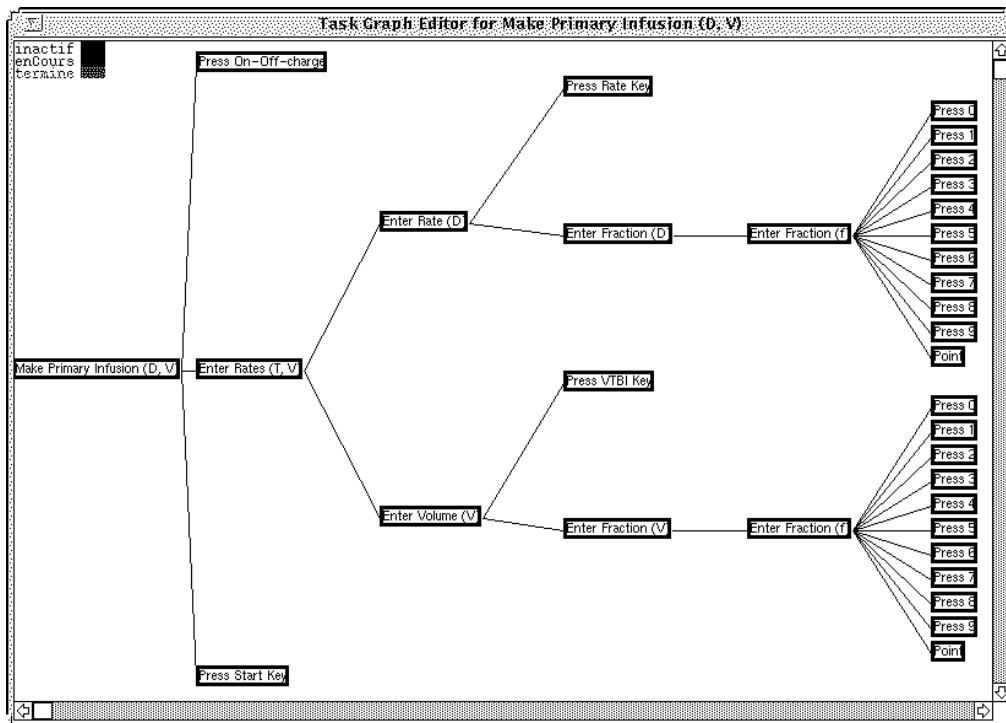
Figure 6. Exemple complet de l'infusion primaire avec fraction.
