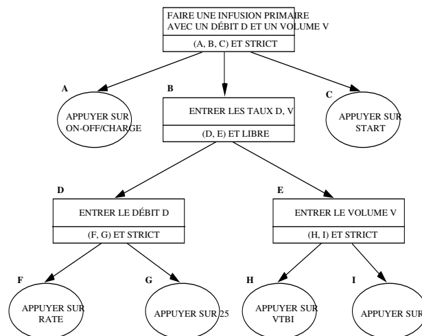
Figure 1. Arbre des tâches pour une infusion primaire avec la pompe Baxter.
