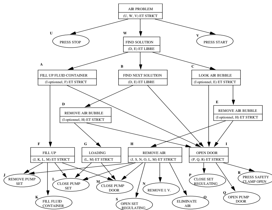
Figure 2. Arbre des tâches pour le problème d'air. Pour des questions de visibilité, le dessin est un graphe, mais la structure sous-jacente est bien un arbre : les noeuds similaires sont dupliqués.
