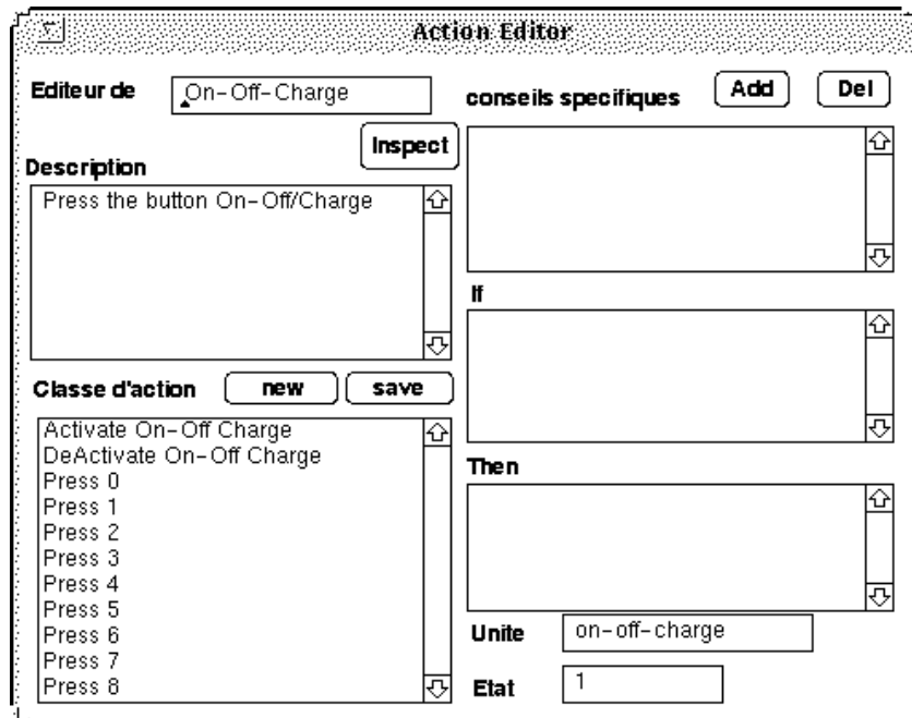
Figure 4: Éditeur d'actions pour le bouton On-Off-Charge.
